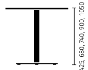
Vaste hoogte met enkele zuil en schotelvoet
