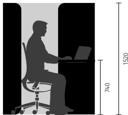
Altura de asiento con pantalla-respaldo
