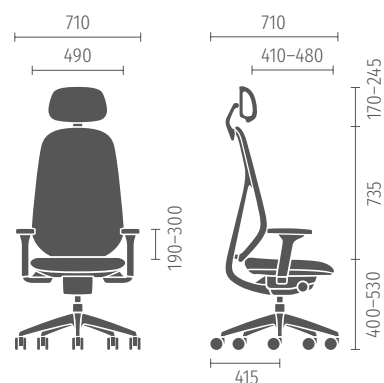
Dossier haut Accoudoirs 4-D et appui-nuque
