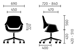
Respaldo bajo
