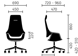
Respaldo alto
