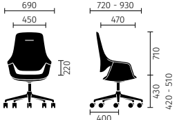
Respaldo medio
