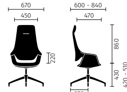
Respaldo alto
