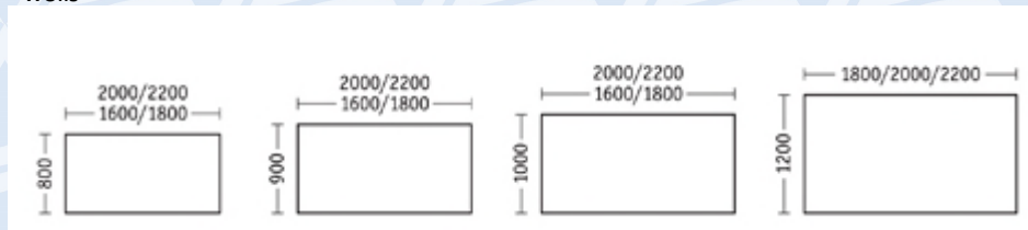
Arbeitstische (optional mit Returntable), Tischhöhe 740 mm
