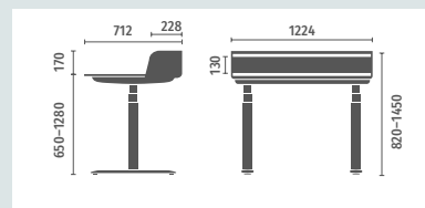
Afmeting tafelblad: B: 1200 x D: 700 mm Afmeting aflegblad: B: 1200 x D: 170 mm
