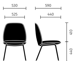
Struttura in acciaio a 4 gambe
