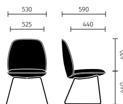
Struttura a slitta
