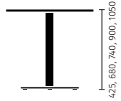
Altezza fissa con colonna singola e base a disco
