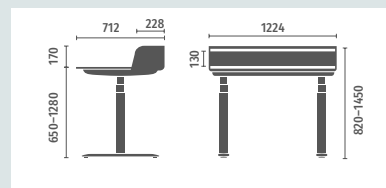
Dimensions du plateau : L : 1200 x P : 700 mm Dimensions de la tablette support : L : 1200 x P : 170 mm
